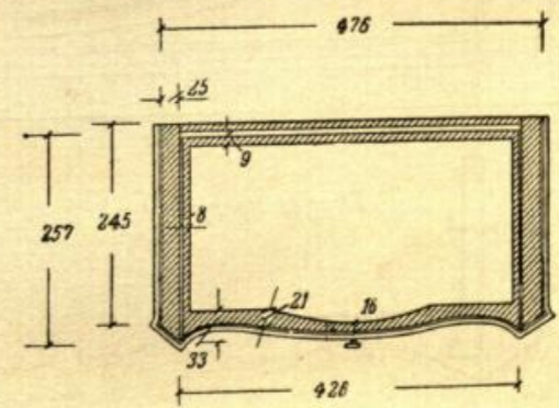
Разрез II-II
