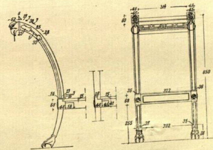
НАЧЕРТЪ 1:4
