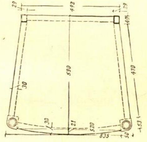
План обвязки (вид сверху)
