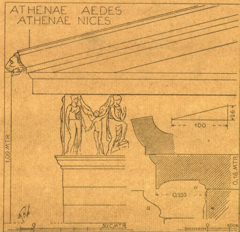
Фиг. 7. Антаблементъ храма Аѣины Побѣды въ Аѣинахъ, по реконструкціи Стівенса.
