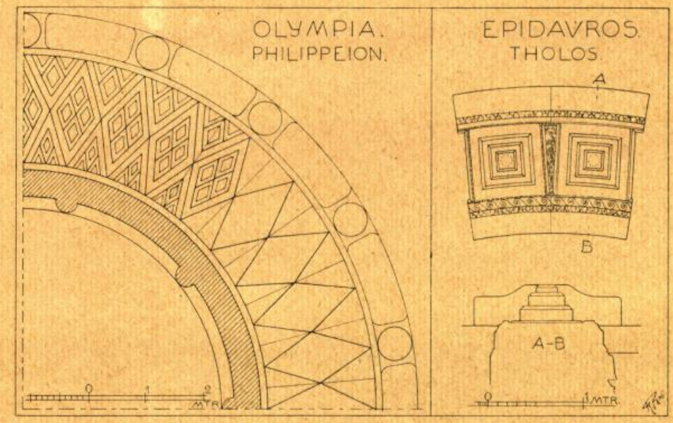
Фиг. 1. Потолокъ наружной колоннады Филиппейона въ Олимпіи. Фиг. 2. Кессонныя плиты внутренней колоннады круглаго зданія въ Эпидаврѣ.
